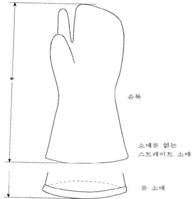
[그림 2] 미트의 모양 ( e:표준길이 )
