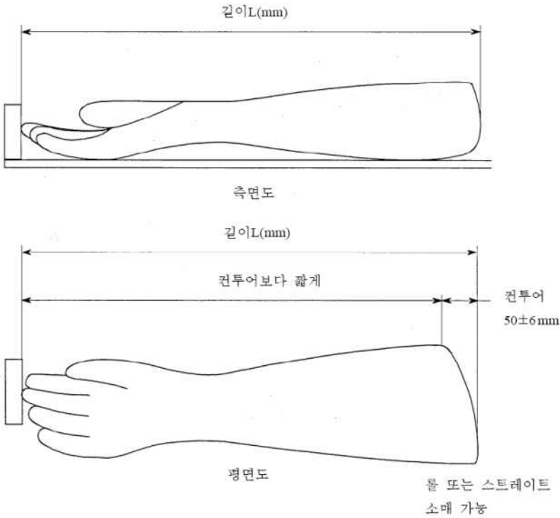
[그림 3] 권투어 장갑의 모양
